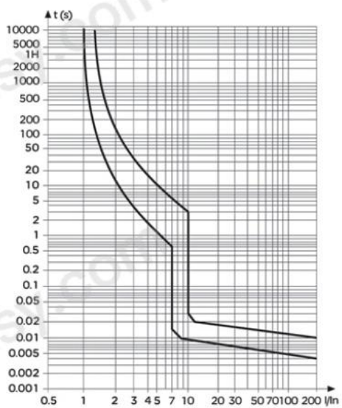
DZ47sZ C型曲线
