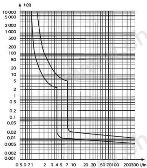
DZ47sZ B型曲线
